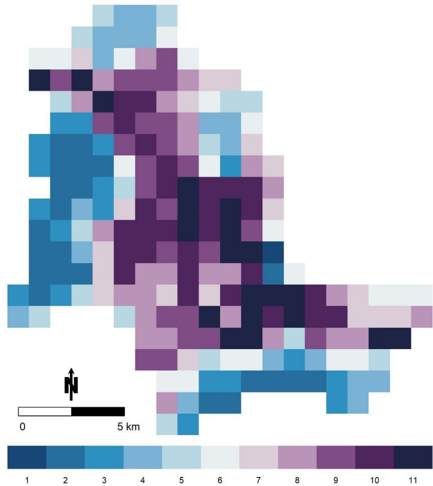
Palermo: Indice di vulnerabilità ambientale e climatica
